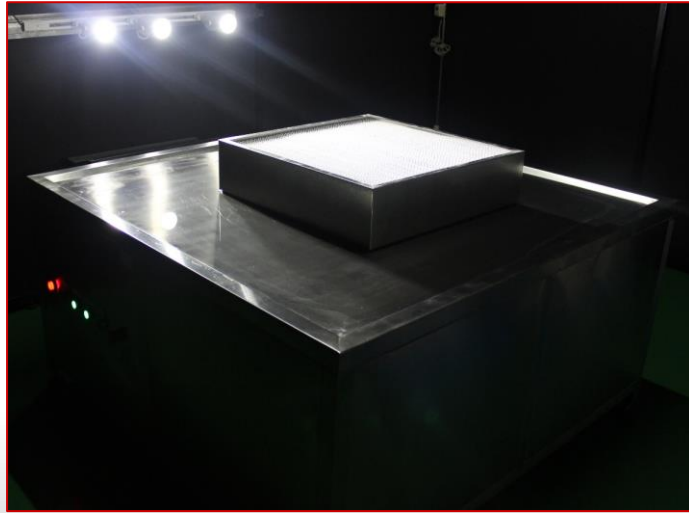
Test độ rò rỉ của lọc Hepa (Smoke Test)
