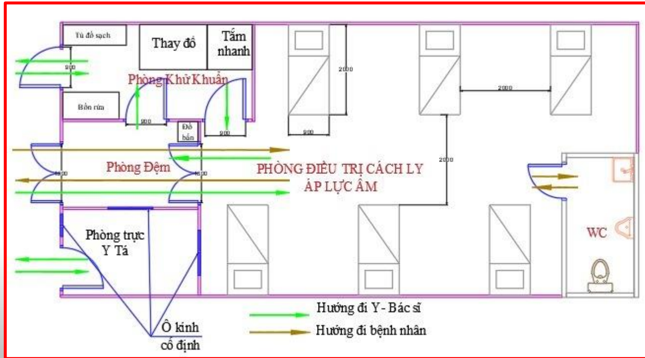
Layout của hệ phòng điều trị cách ly áp lực âm đặc trưng
