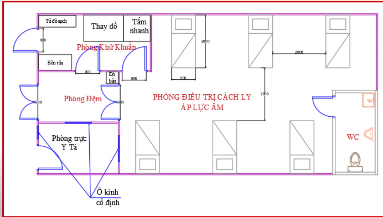
Layout của hệ phòng điều trị cách ly áp lực âm đặc trưng
