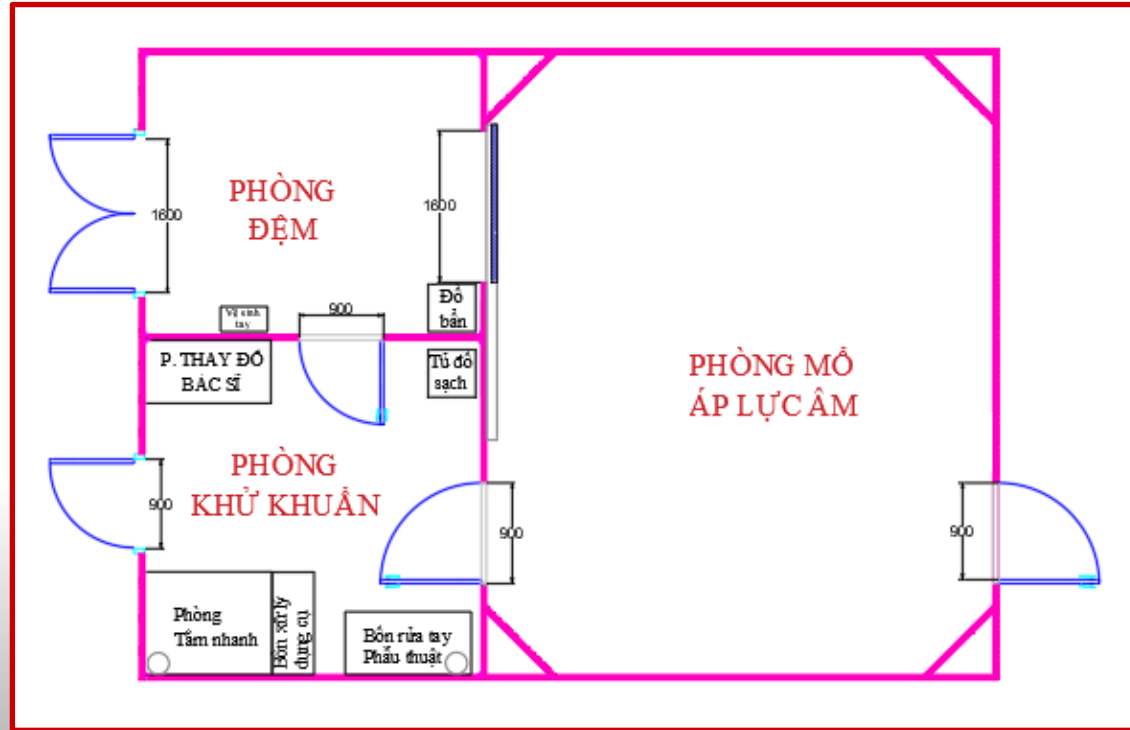
Layout của hệ phòng mổ áp lực âm đặc trưng
